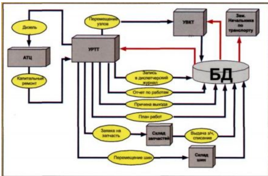
Рис. 1. Взаимодействие в АСУ ТОиР "TRIM": эксплуатация автосамосвалов
