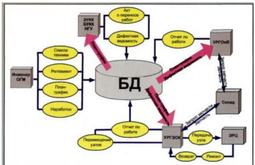
Рис. 2. Взаимодействие в АСУ ТОиР "TRIM": ремонт автосамосвалов
